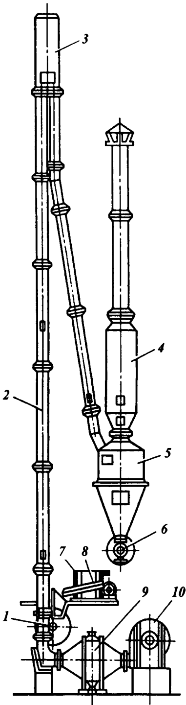
Рис. X-16. Схема пневматической сушилки: 1 — питатель; 2 — сушильная труба; 3 — сборник; 4 — фильтр; 5 — циклон; 6 — выгрузатель; 7 — бункер влажного материала; 8 — дозатор; 9 — воздухоподогреватель; 10 — вентилятор
